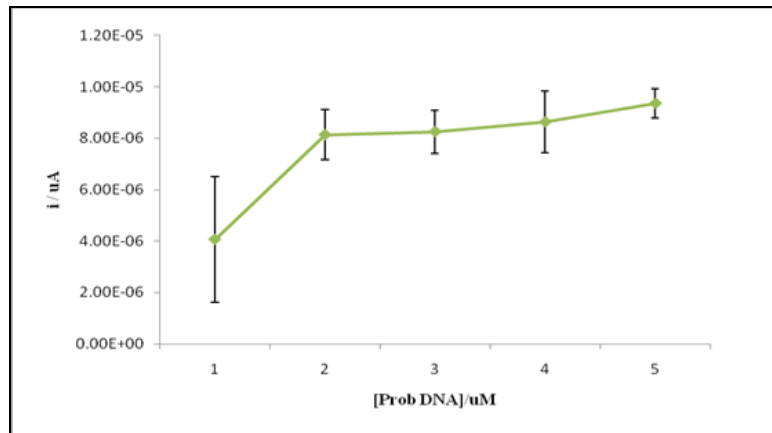
Rajah 5. Kesan kepekatan prob DNA terhadap rangsangan biosensor DNA. Penghibridan dilakukan dalam larutan penimbal Na-fosfat 0.05 M pada pH 7.0 yang mengandungi 1 M NaCl dan [\text{Ru}(\text{bpy})_2\text{PIP}]^{2+}
